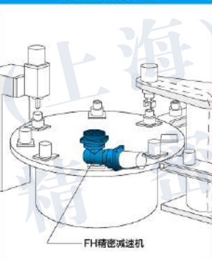
分度工作台驱动
