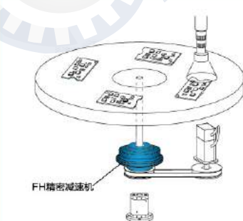
印刷电路板检查装置
