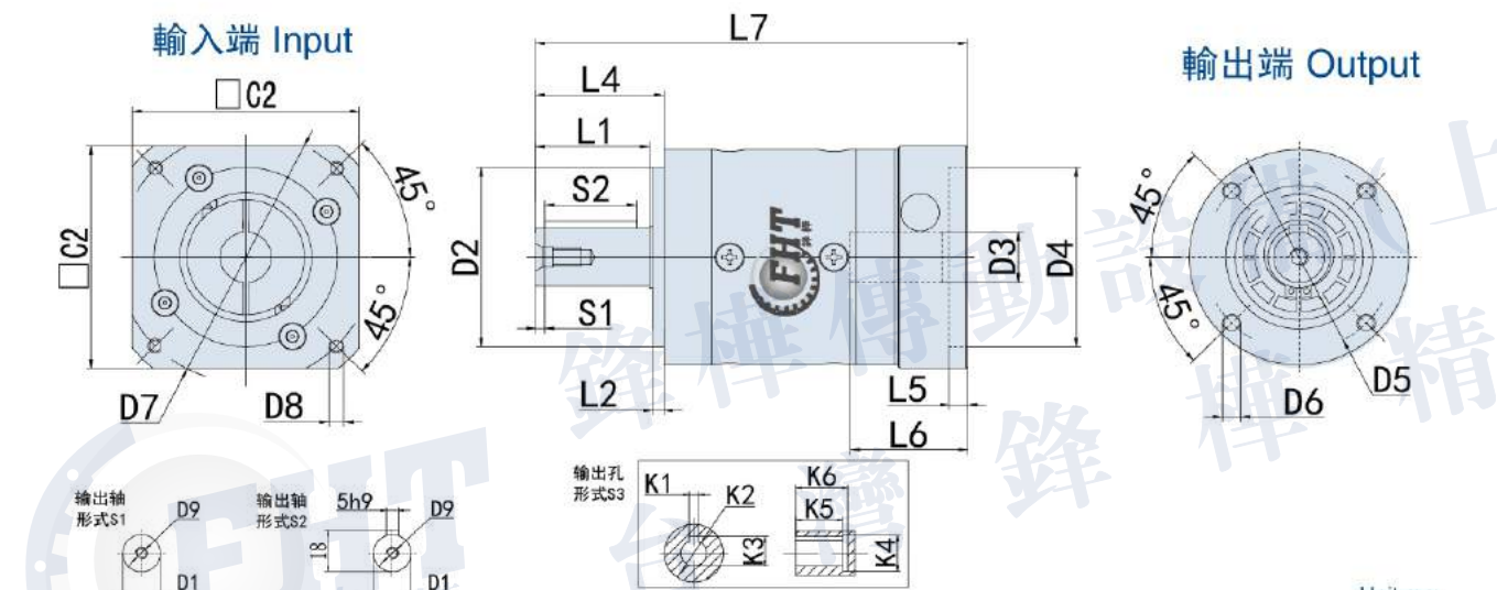
外形尺寸圖 Dimensions:
