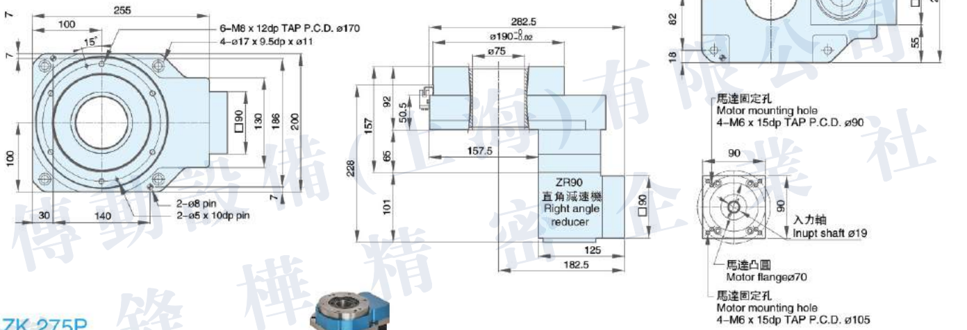
ZK 275R (直角轉向式1:20)
