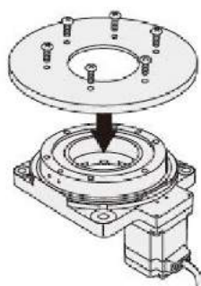
DGII系列 (一体化产品)
