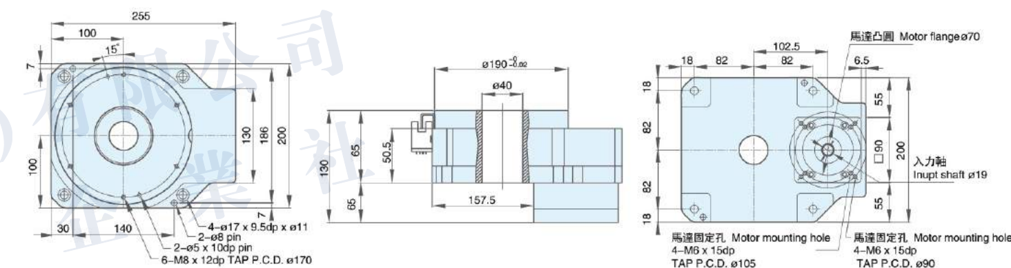
ZK 200 (附連接座可自行組裝馬達)
