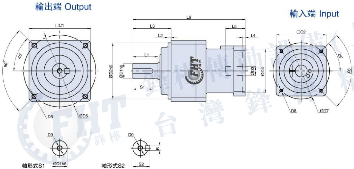
外形尺寸圖 Dimensions:
