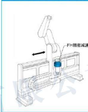
机器人的行走轴(齿条&小齿轮)
