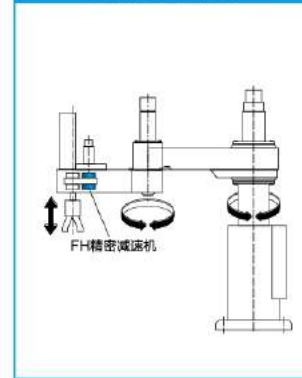
水平多关节机器人
