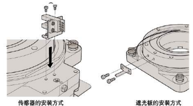
傳感器的安裝方式
