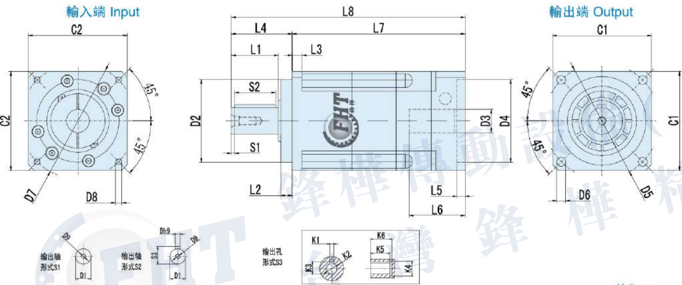
外形尺寸圖 Dimensions:
