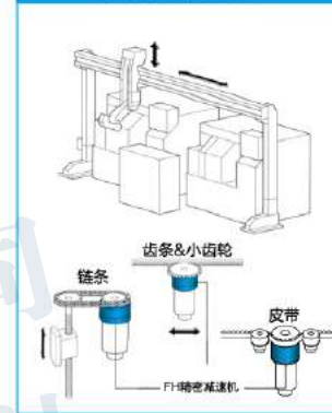
机床的龙门机器人
