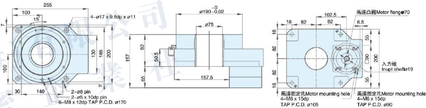
ZK 275 (附連接座可自行組裝馬達)
