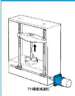
拉力试验机
