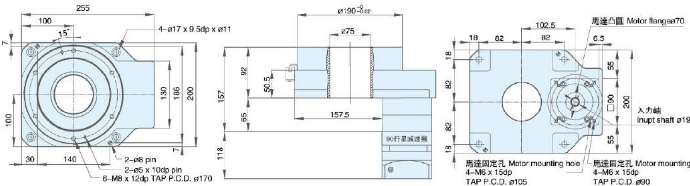
ZK 275P (附行星減速機速比 30,40,50)
