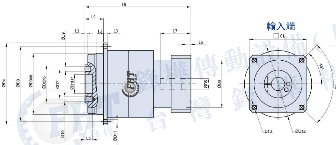
外形尺寸圖 Dimensions:
