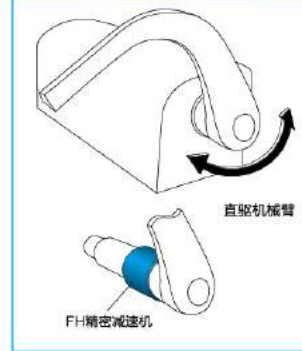
注塑成型取出机器人
